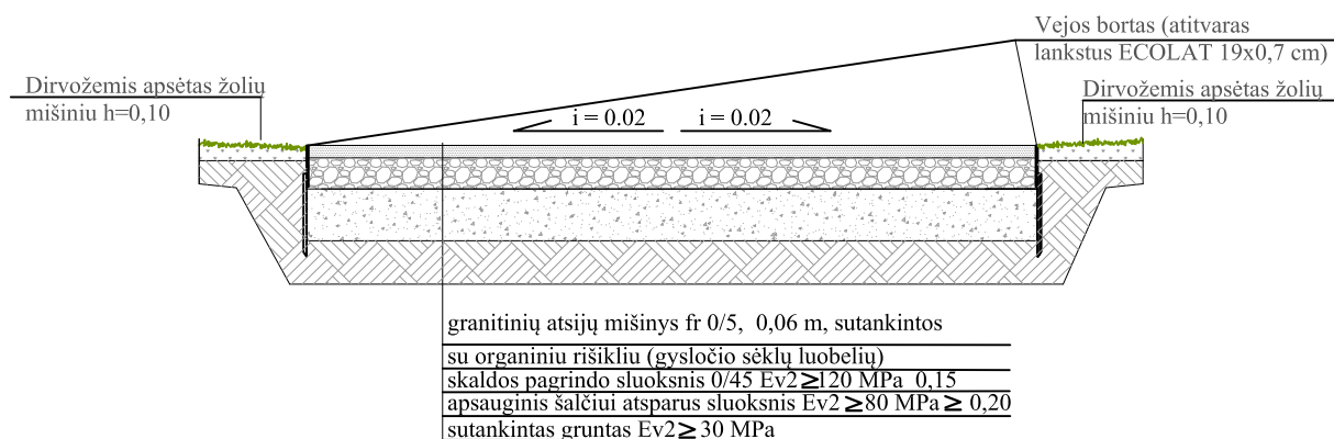
Skersinis gruntinio tako su vejos borto pjūvis
