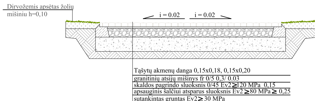
Skersinis tašytų akmenų dangos tako pjūvis
