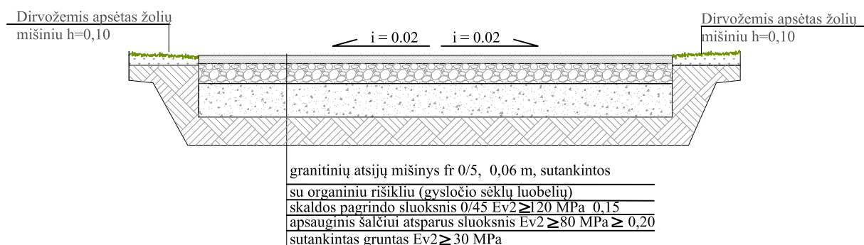
Skersinis gruntinio tako be borto pjūvis
